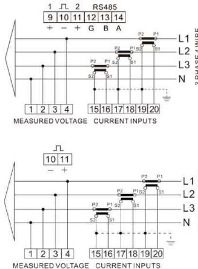
SDM72CT-M
